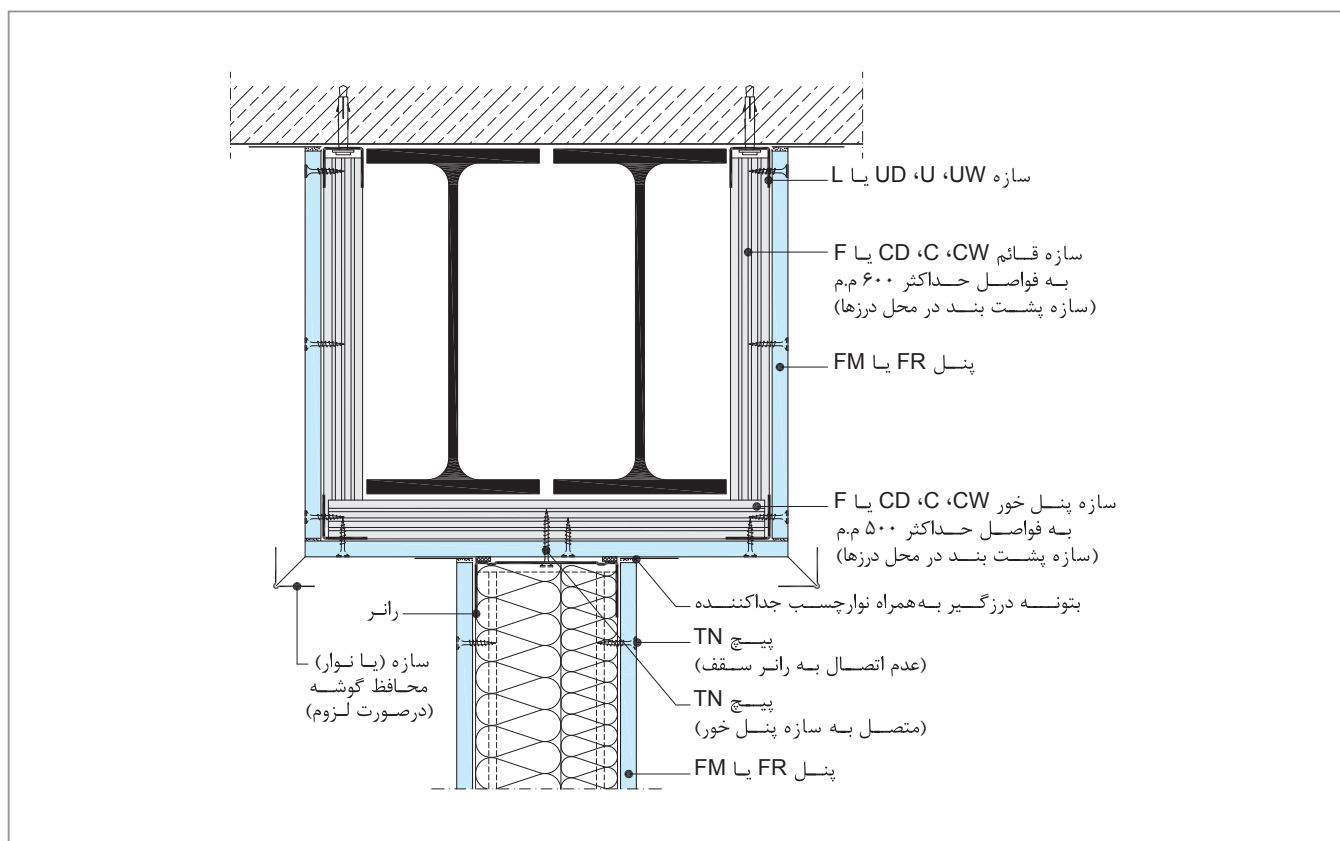
اتصال دیوار خشک به پوشش محافظ تیر (ثابت)
