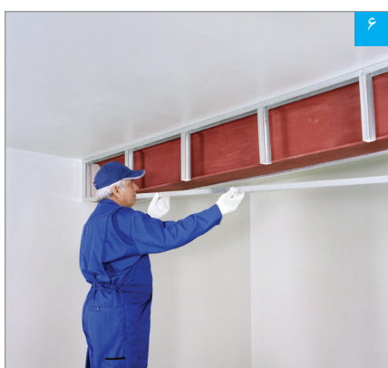
۶ استقرار سازه تحتانی
