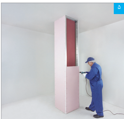
اجرای پنل‌های لایه اول
