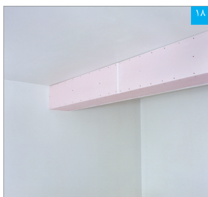
پوشش محافظ تیر تکمیل شده
