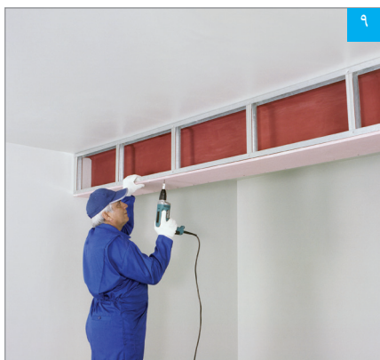
۹ اجرای پنل تحتانی
