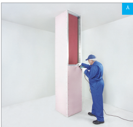
ایجاد اتصال میان سازه پشت بند درز و پنل
