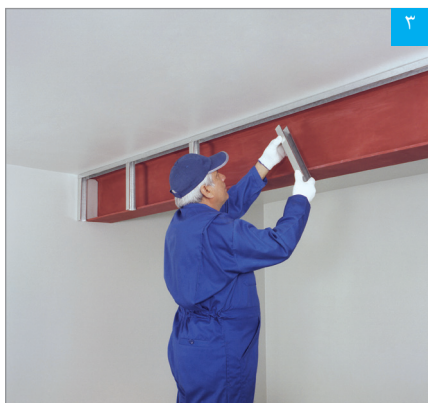
۳ اجرای سازه‌های قائم
