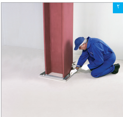
اتصال رانرها
