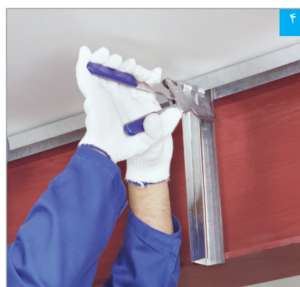
۴ اتصال سازه‌های قائم به سازه فوقانی (با استفاده از پانچ)
