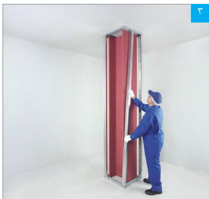
استقرار استاداها در رانرهای کف و سقف
